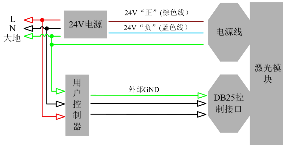
图 4 电气连接图
