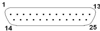
图 5 控制接口图
